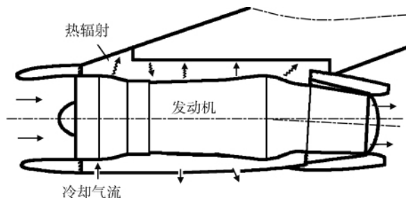
图2 短舱冷却系统的工作原理
