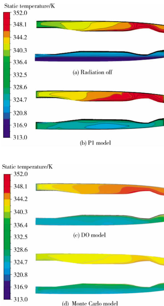
图 5 不同辐射模型的对称面温度分布
