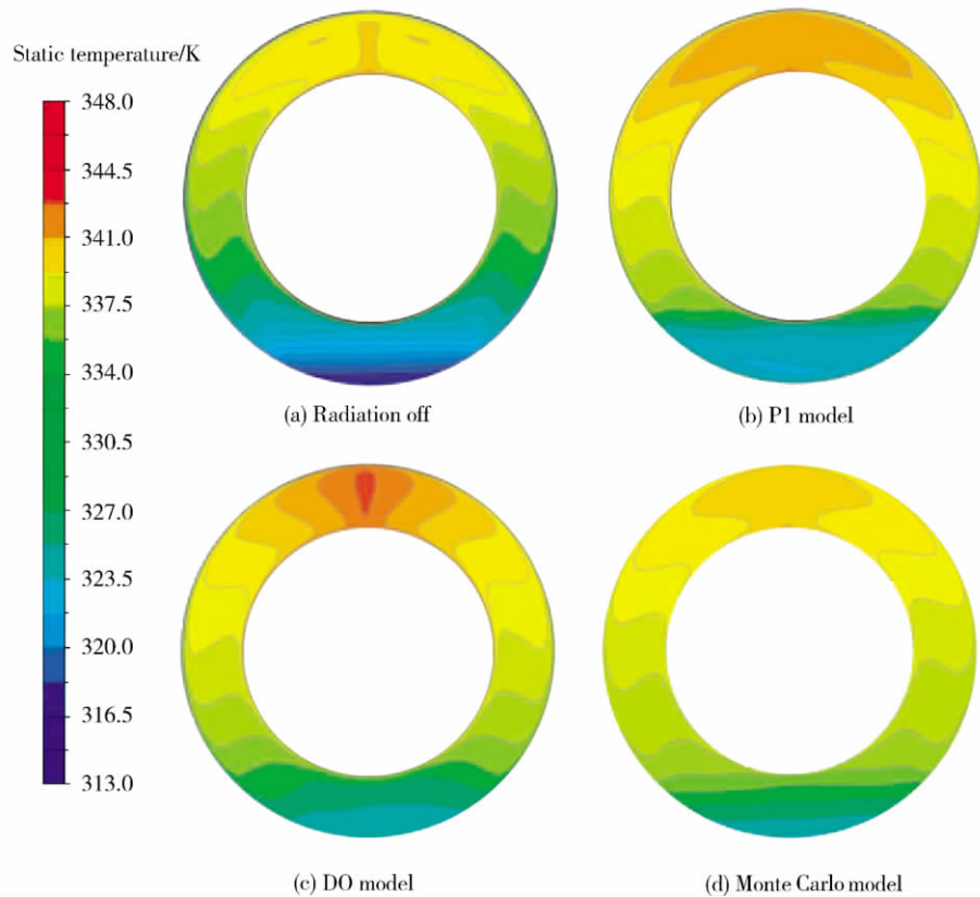
图 6 不同辐射模型的计算截面温度分布
