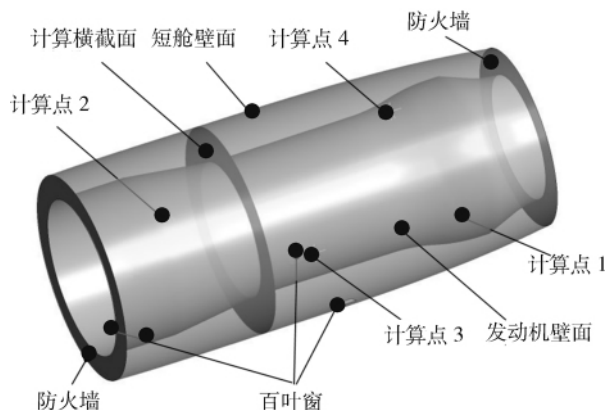
图3 计算模型及计算点/截面位置
